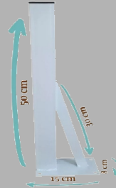
MÃO FRANCESA PARA FIXAÇÃO DE BANCADAS (REFORÇADA) METALON 50X30
